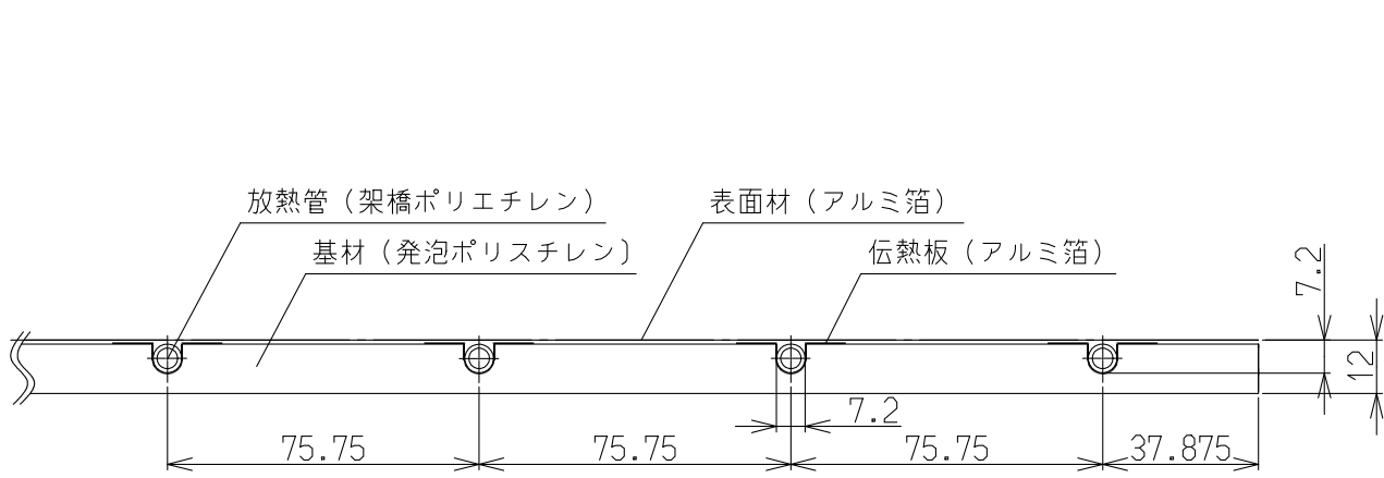
(A-A'断面図)
