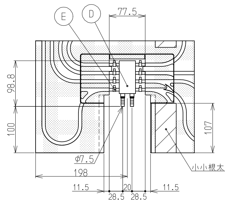
ヘッダー部詳細図
