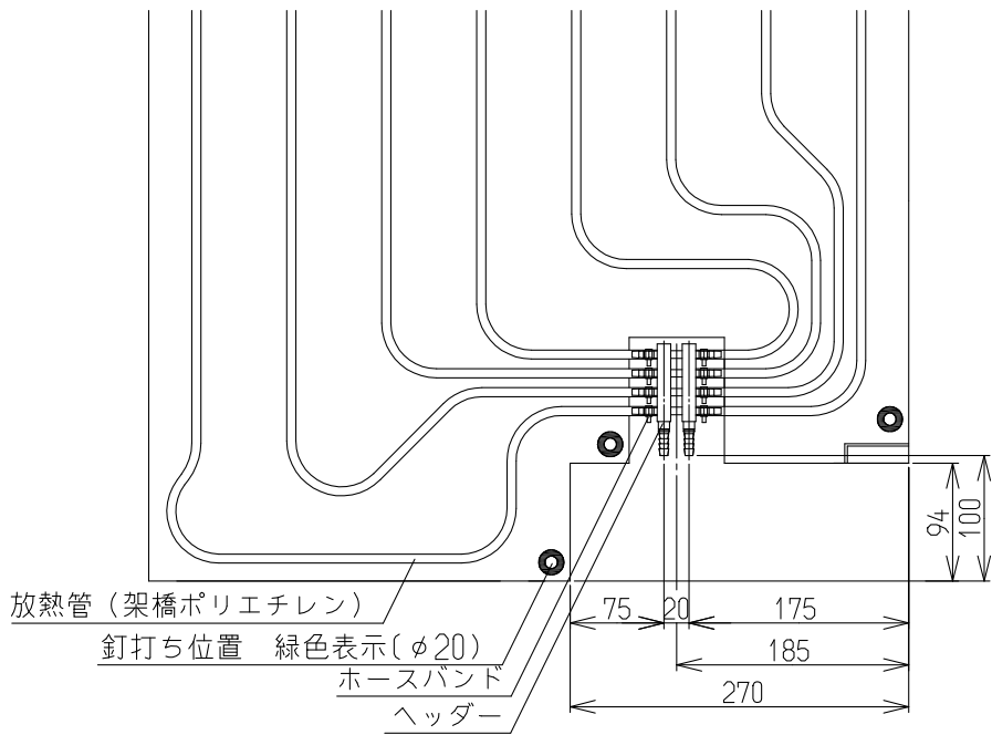
ヘッダー部拡大図
