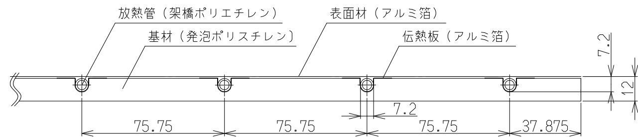
(A-A'断面図)
