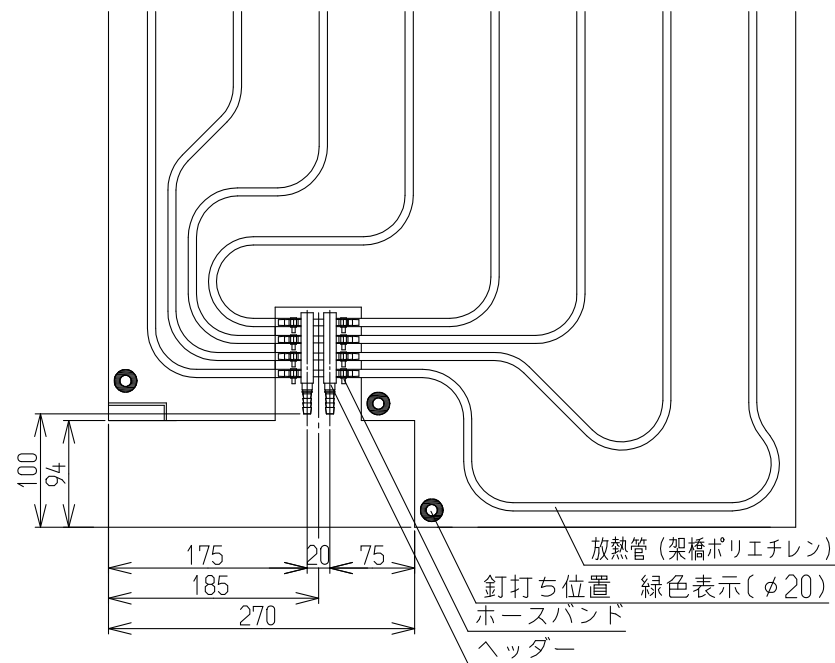
ヘッダー部拡大図
