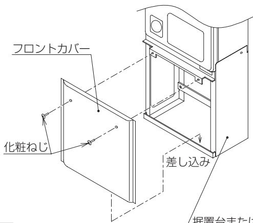
<①フロントカバーのはずしかた・取り付けかた>
