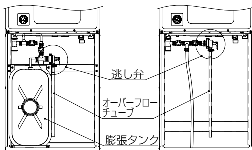
膨張タンクがある場合
