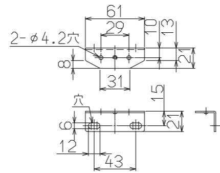
取付金具下(左右共通) 尺度:フリー
