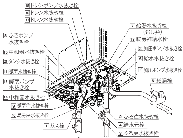
熱動弁内蔵タイプ
