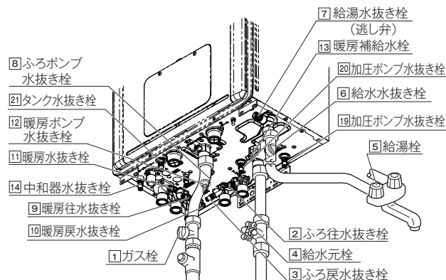
熱動弁外付けタイプ
