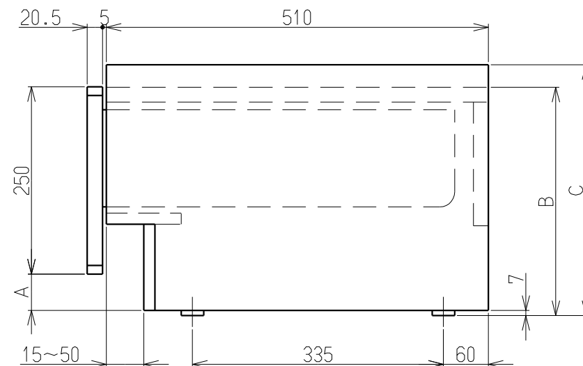
側面図
