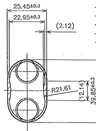
A-A断面图
