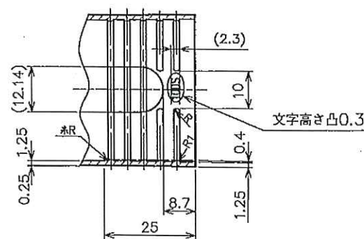
C-C断面图
