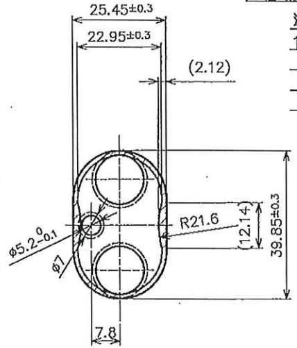
A-A断面図
