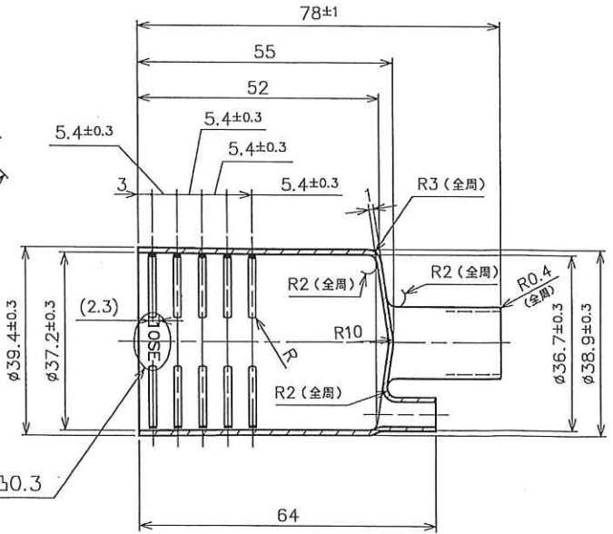
A-A断面図
