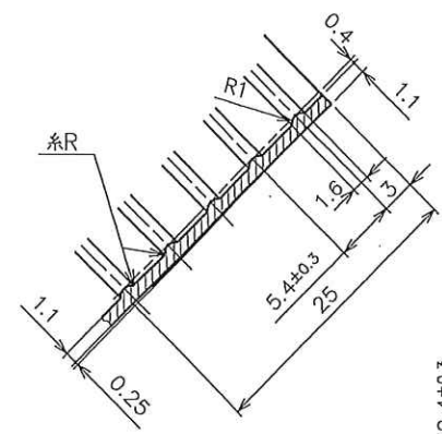
B-B断面図 (S=2:1)
