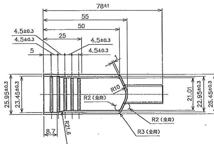
B-B断面图
