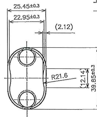
A-A断面图
