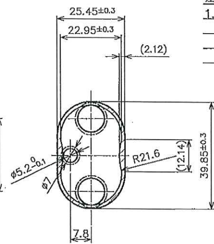
A-A断面図
