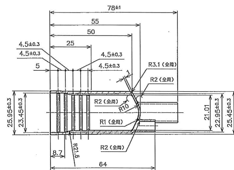
B-B断面図
