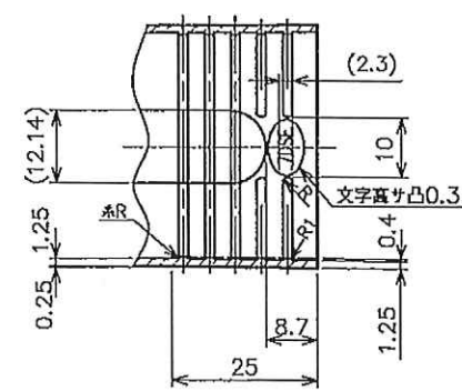
C-C断面図
