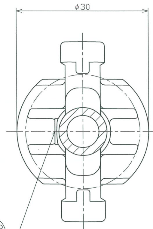
B-B断面
