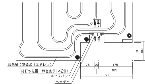
ヘッダー部拡大図
