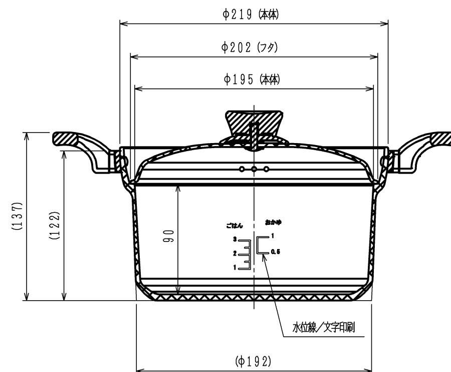
AA断面図
