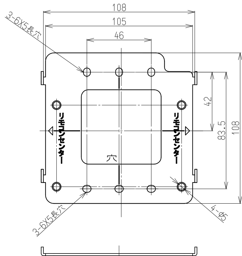
リモコン壁取付金具 t=1.6
