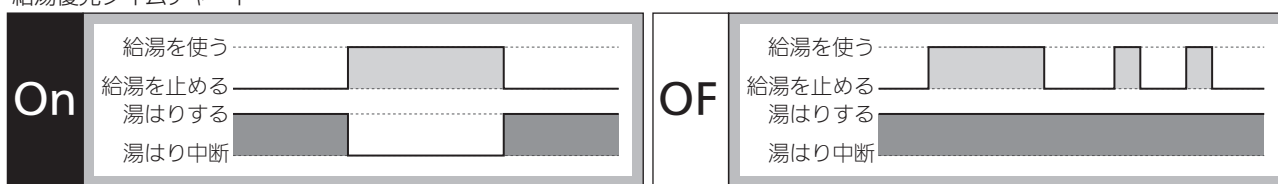
給湯優先タイムチャート
