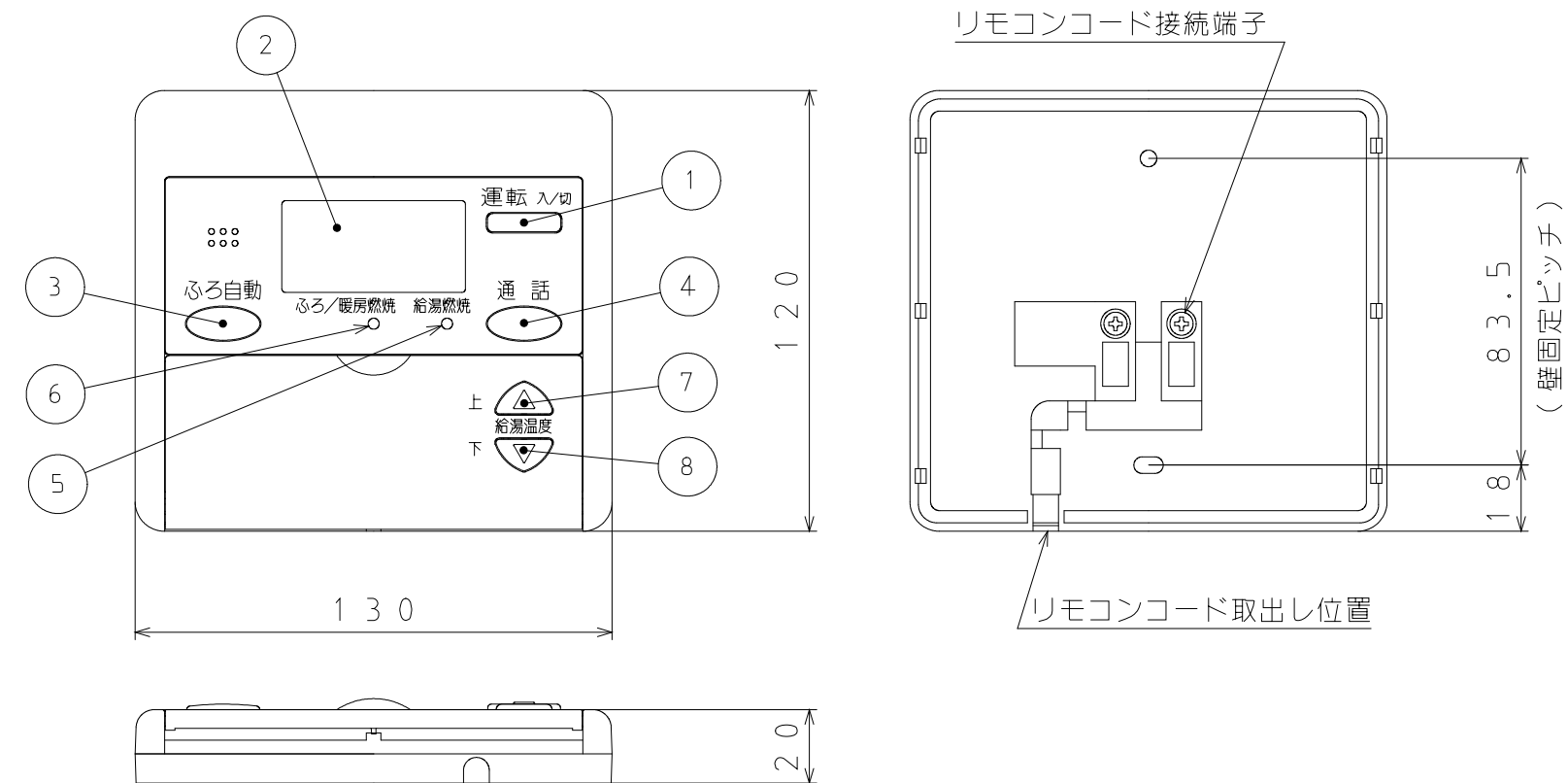
◎ MC-637 (暖房SW付) ふたを開いた状態
