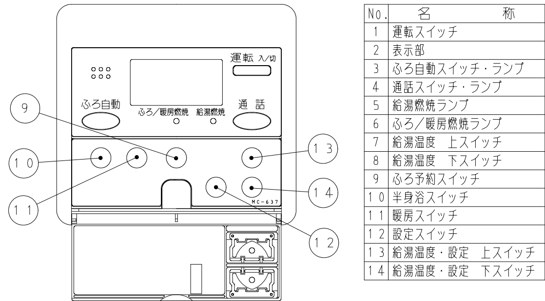
◎ MC-637 (暖房SW付) ふたを開いた状態
