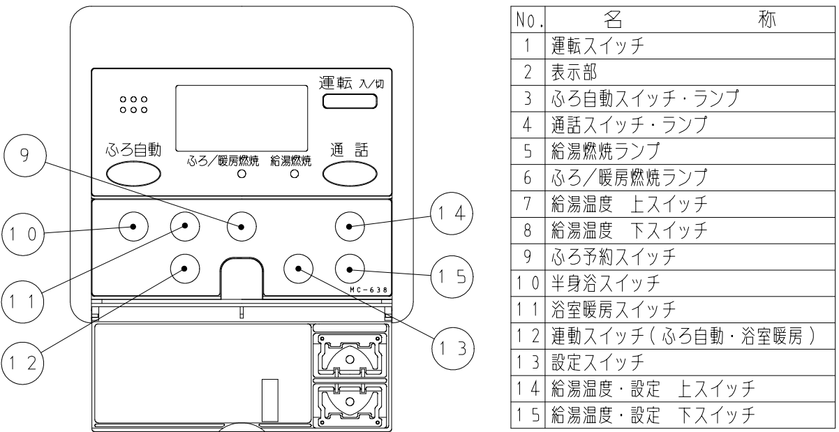
◎ MC-638 (浴室暖房SW付) ふたを開いた状態
