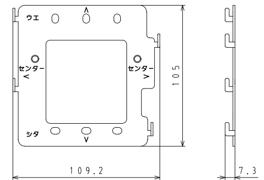
壁取付金具 寸法図
