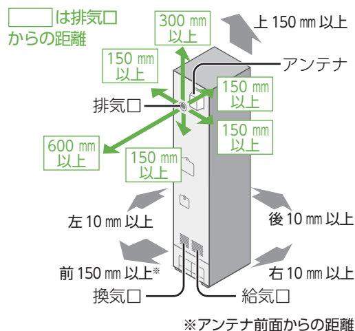
貯湯ユニット
