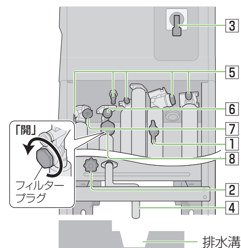
貯湯ユニットの内側
