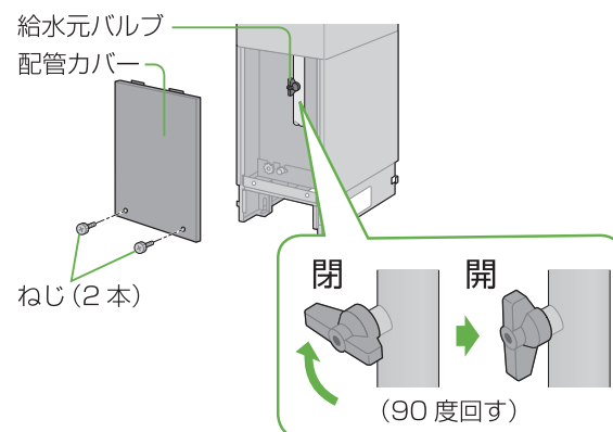
貯湯ユニット
