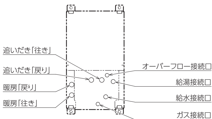
配管位置図
