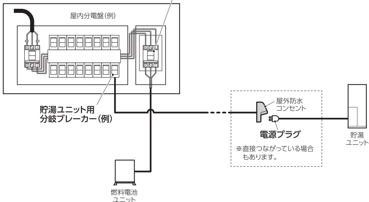
燃料電池ユニット用専用ブレーカー（例）
