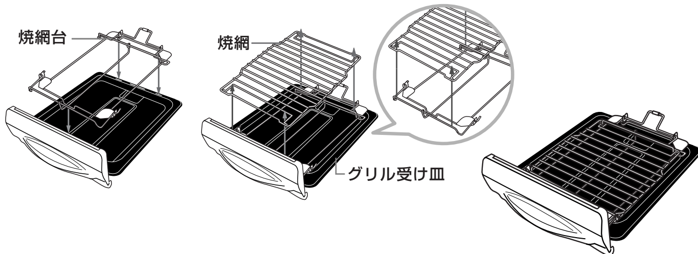
組立図
