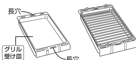
【組立図】
