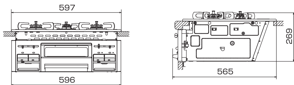
外形寸法図 (単位:mm)
