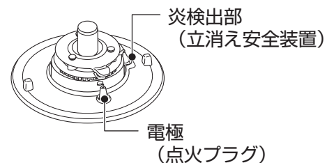
小バーナ
