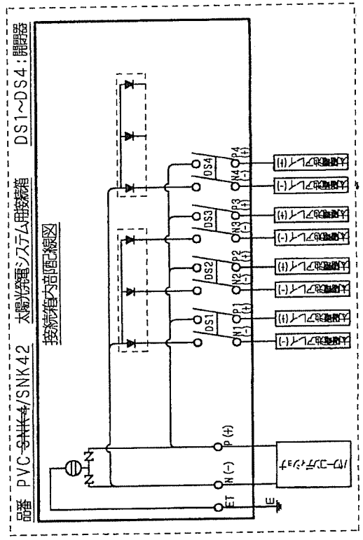
PVC-SNK4/SNK42 回路図(4回路)
