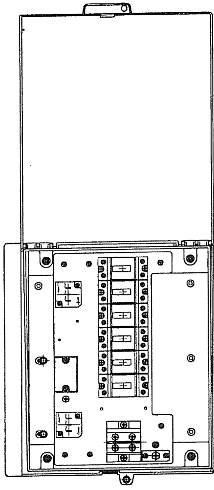
PVC-SNKG/SNK62 内部図(6回路)
