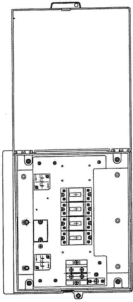
PVC-SNK4/SNK42 内部図(4回路)
