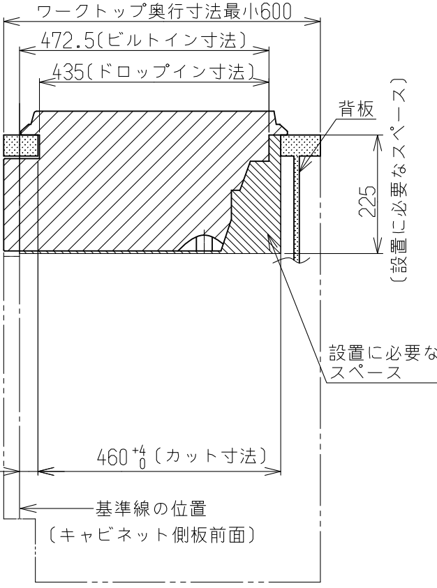
側面図
