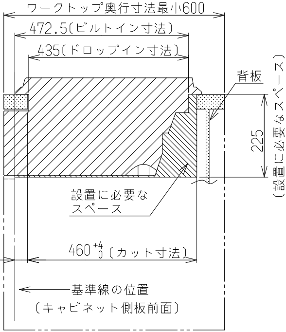
側面図
