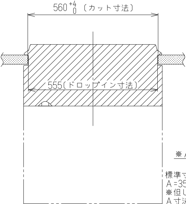
正面図
