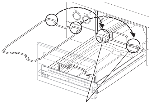
プレート固定枠をここにのせる
