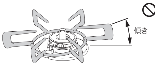
誤った取り付けの例
