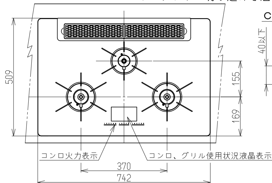
ワークトップ切り込み寸法
