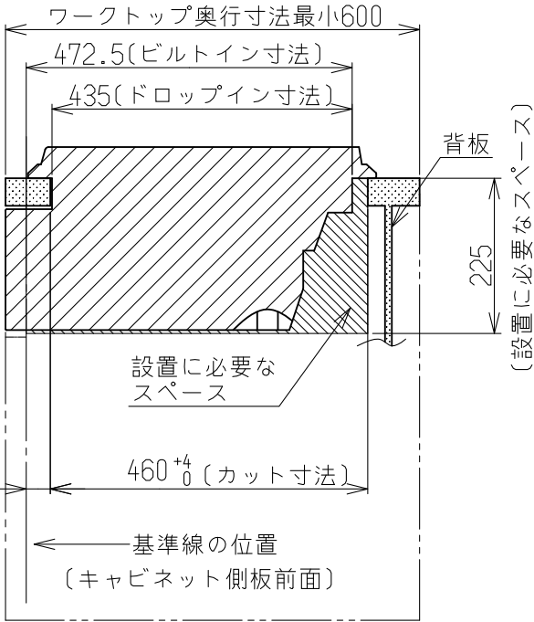
側面図
