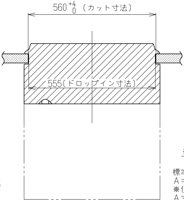
正面図
