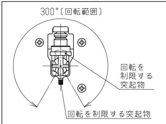
ガス接続口の回転範囲
