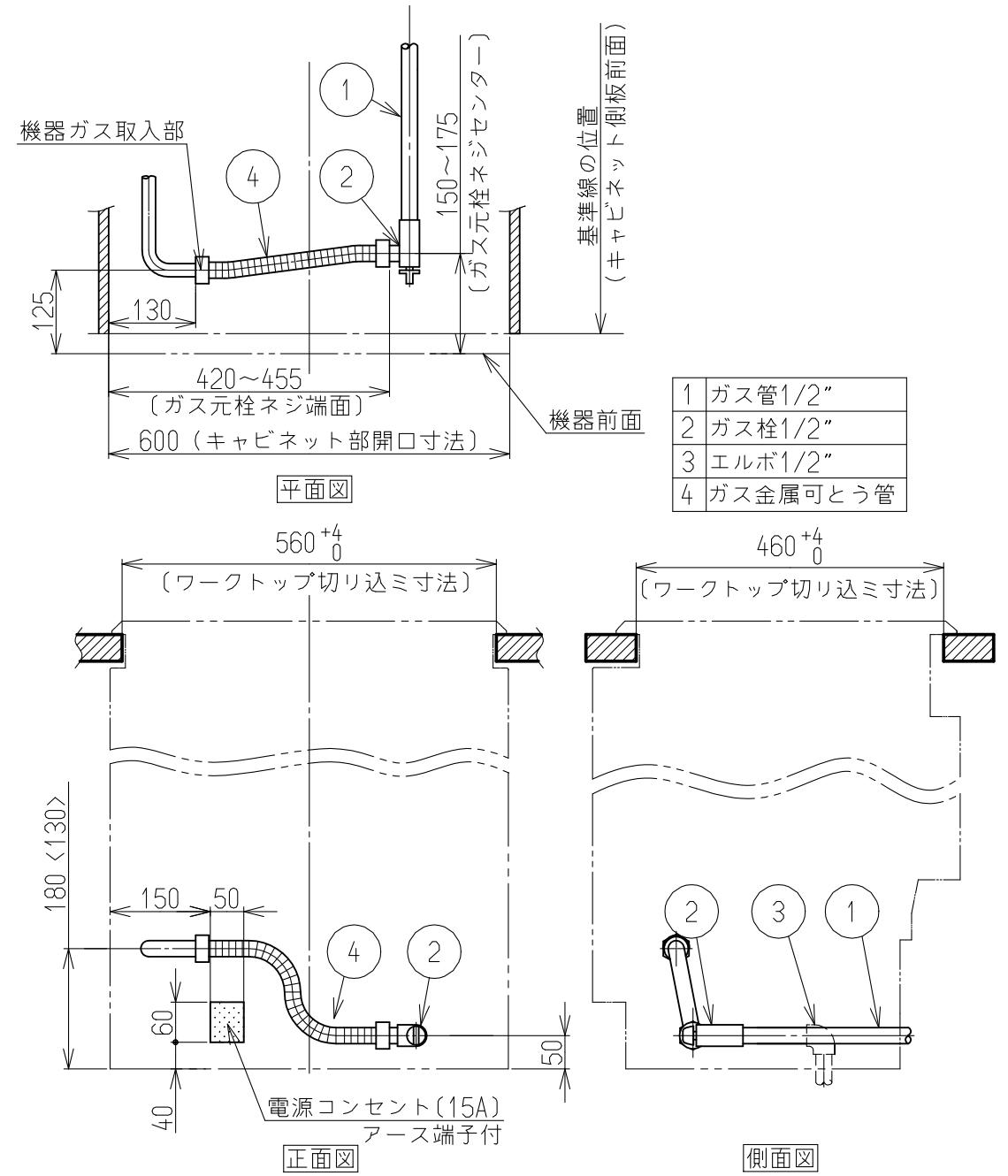
配管施工例図(尺度:F)
