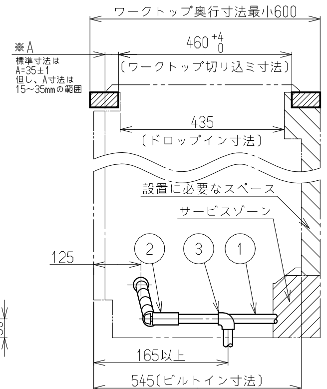
設置・配管施工例図
