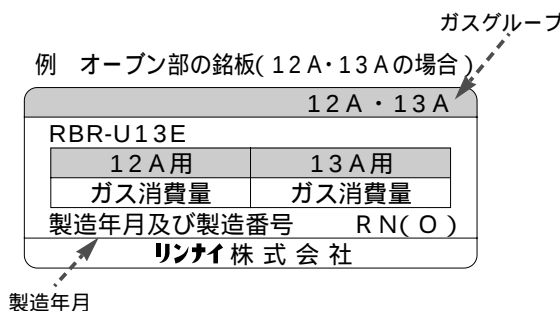
例 銘板
