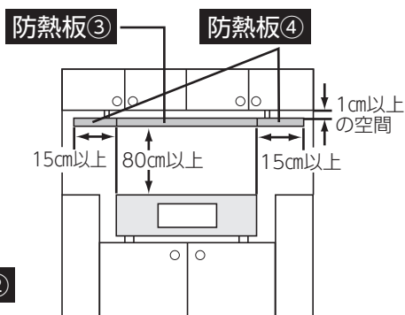
上 面
