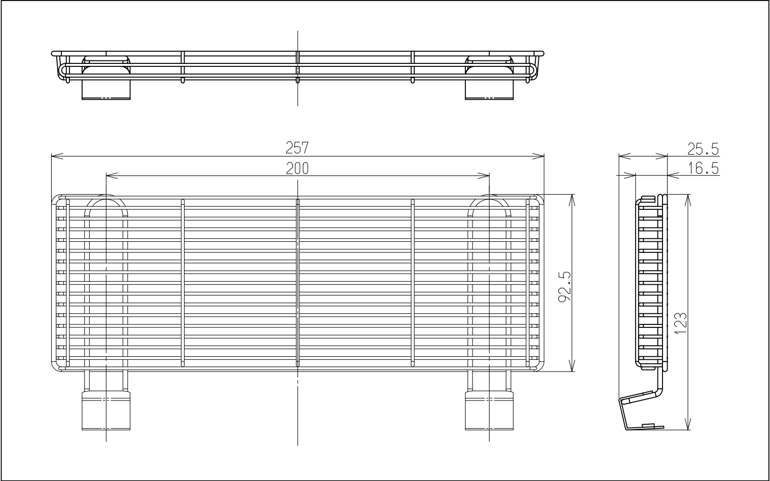
グリル扉ガード本体 寸法図 (1:2)
