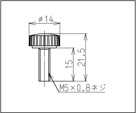
固定用ネジ 寸法図 (1:1)
