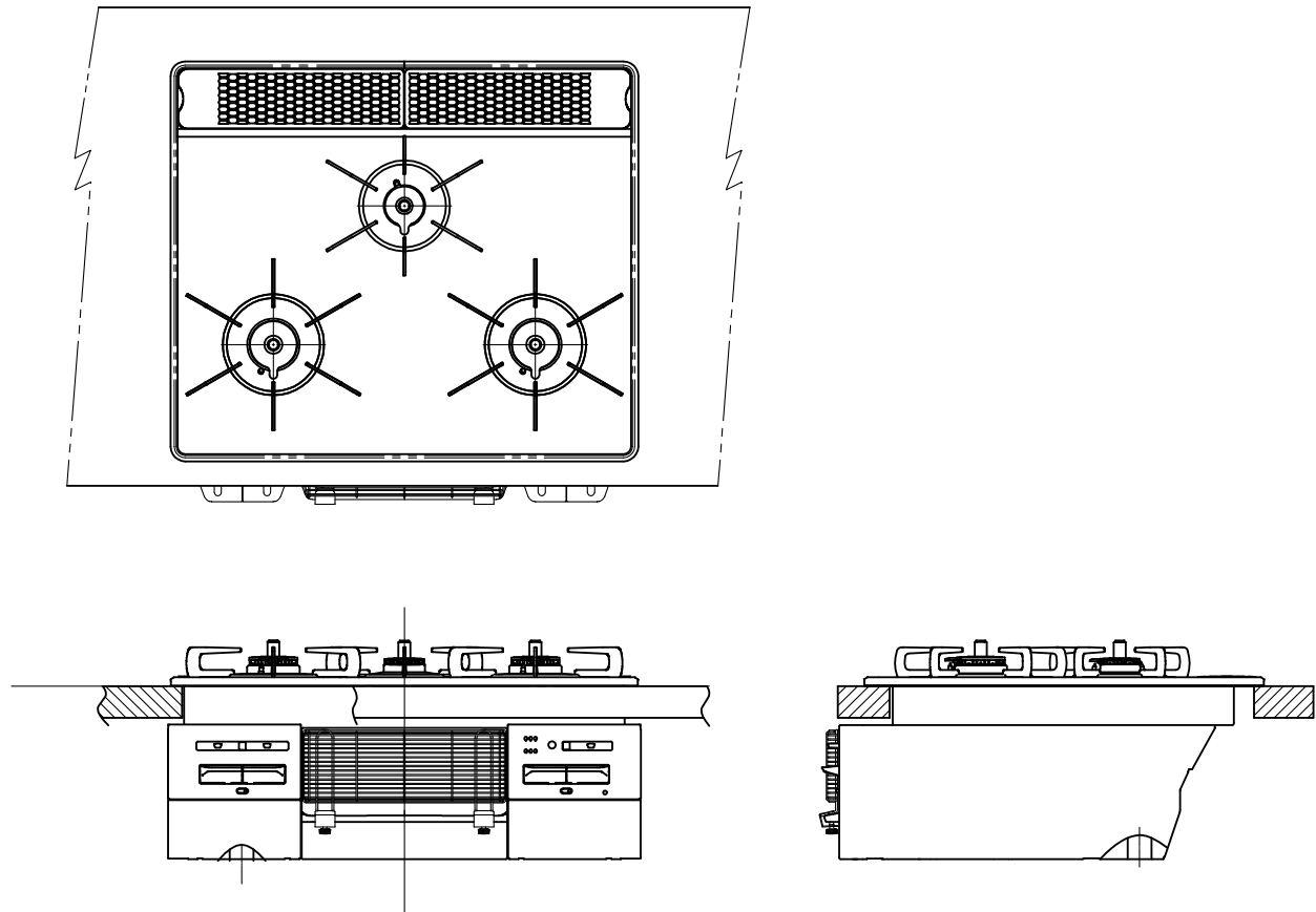
設置図
