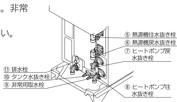
タンクユニット水抜き栓詳細図
