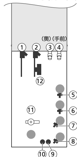
タンクユニット水抜き栓概要図
