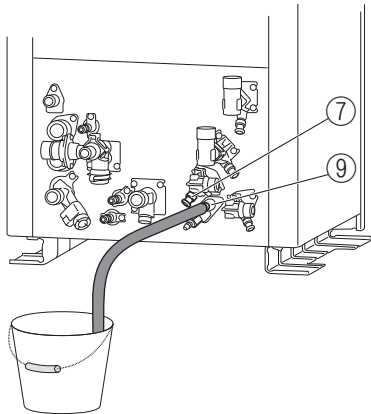
RTU-R505(S)-U、RTUP-R506(S) の場合
