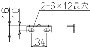
取付金具下(左右共通) 尺度：フリー
