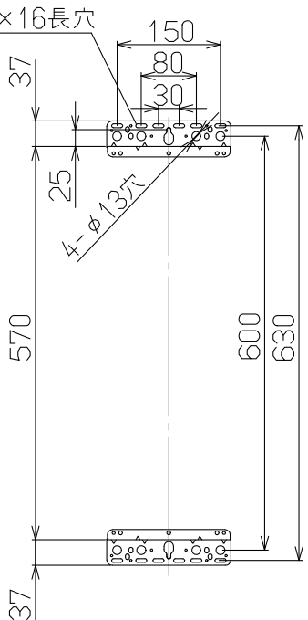
壁掛金具
