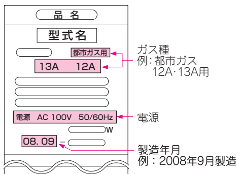
銘板例
