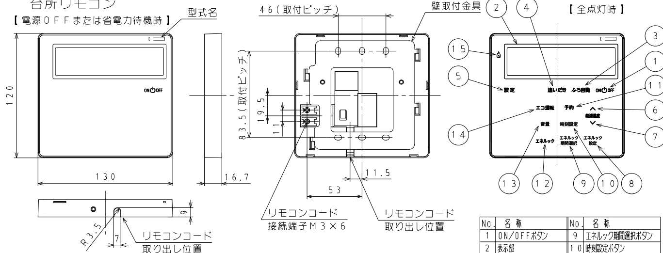
壁取付金具 寸法図
