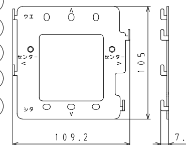
壁取付金具 寸法図
