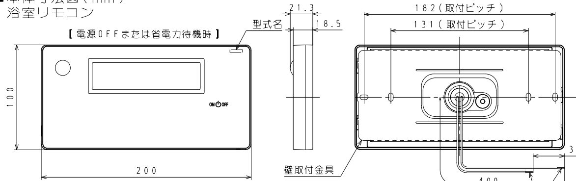
壁取付金具 寸法図 材質: SUS304 板厚: t1.0
