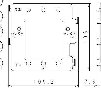
壁取付金具 寸法図 材質: L50 板厚: t1.6
