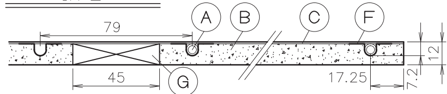
A-A' 詳細図 1 / 2
