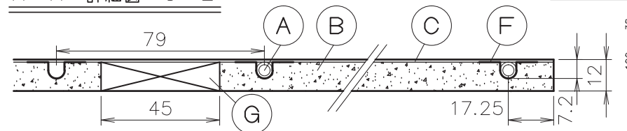
A-A' 詳細図 1 / 2
