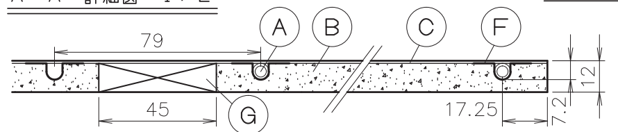
A-A' 詳細図 1 / 2
