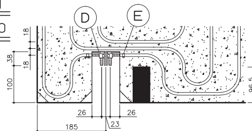
ヘッダー部詳細図
