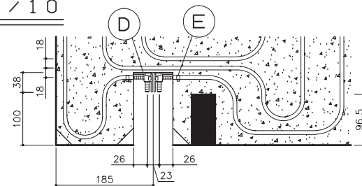
ヘッダー部詳細図
